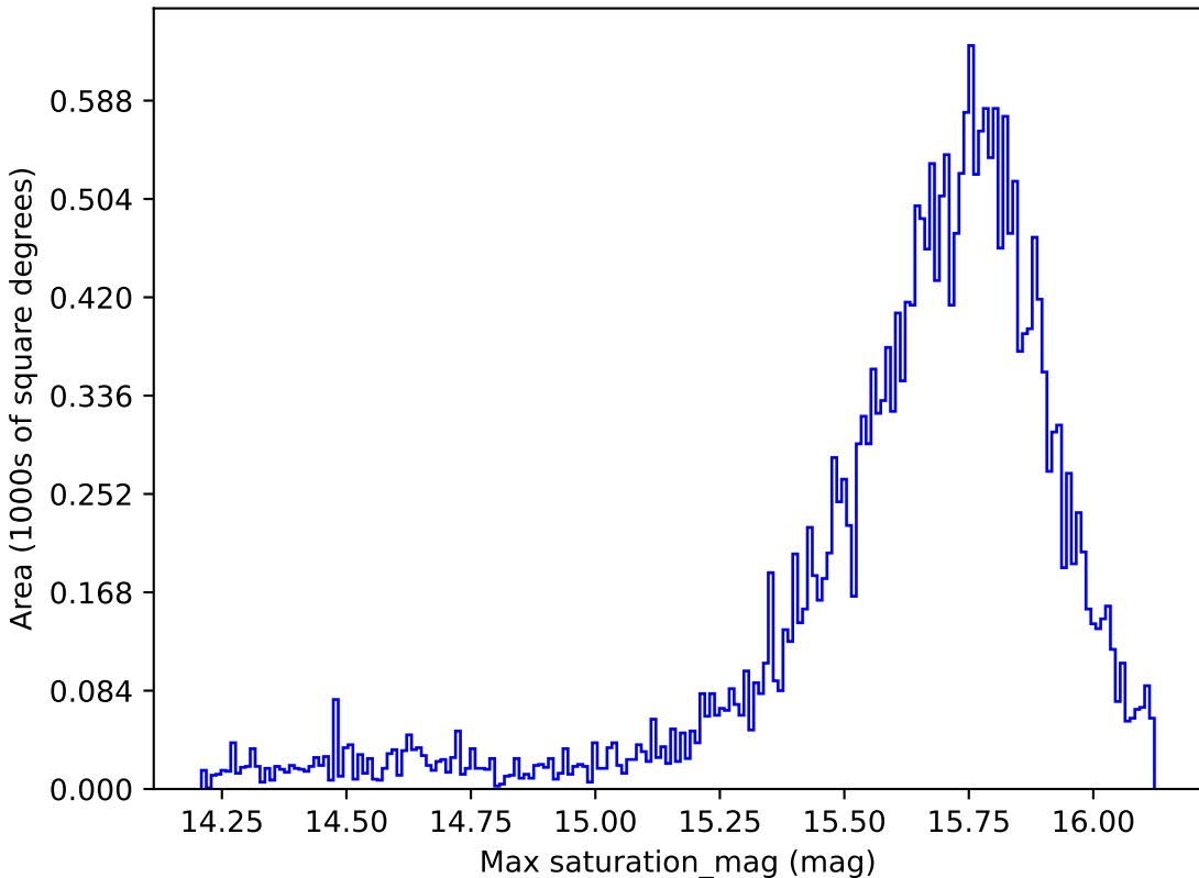
baseline_v3.3_10yrs All sky g band: Max saturation_mag
