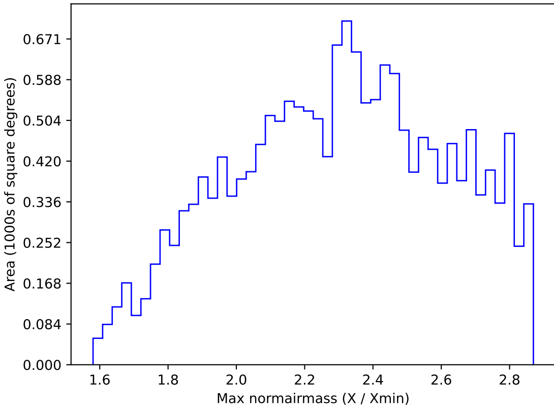
baseline_v3.3_10yrs WFD z band: Max normairmass
