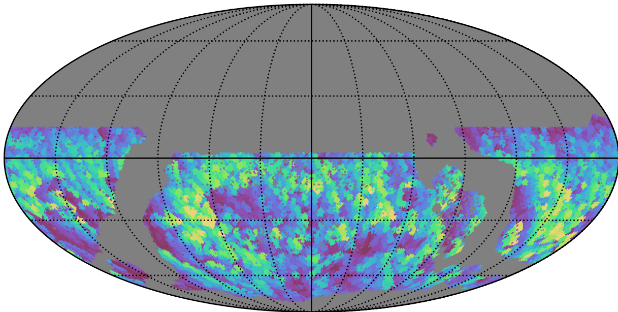
baseline_v3.3_10yrs WFD y band: Max normairmass
