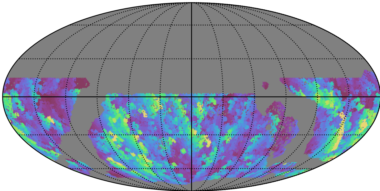
baseline_v3.3_10yrs WFD u band: Max normairmass
