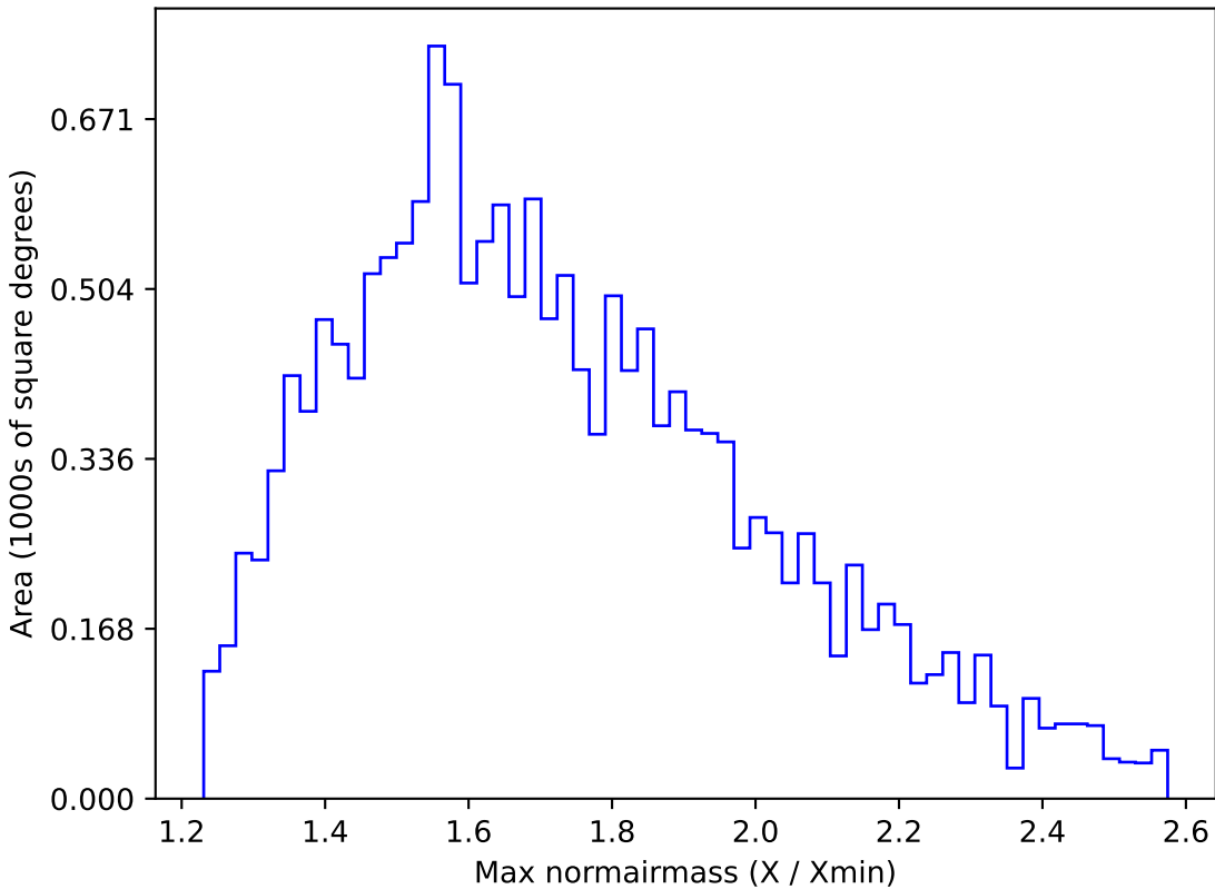
baseline_v3.3_10yrs WFD u band: Max normairmass
