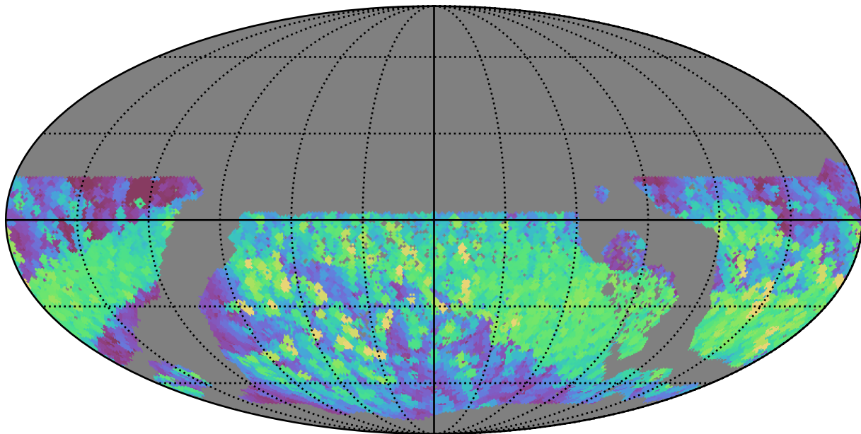
baseline_v3.3_10yrs WFD r band: Max normairmass
