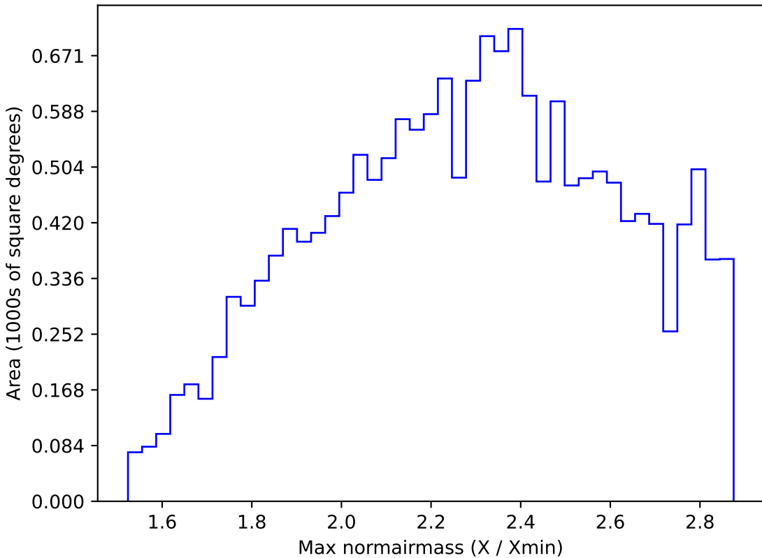
baseline_v3.3_10yrs WFD i band: Max normairmass
