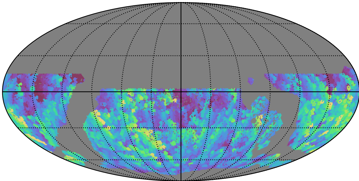
baseline_v3.3_10yrs WFD g band: Max normairmass
