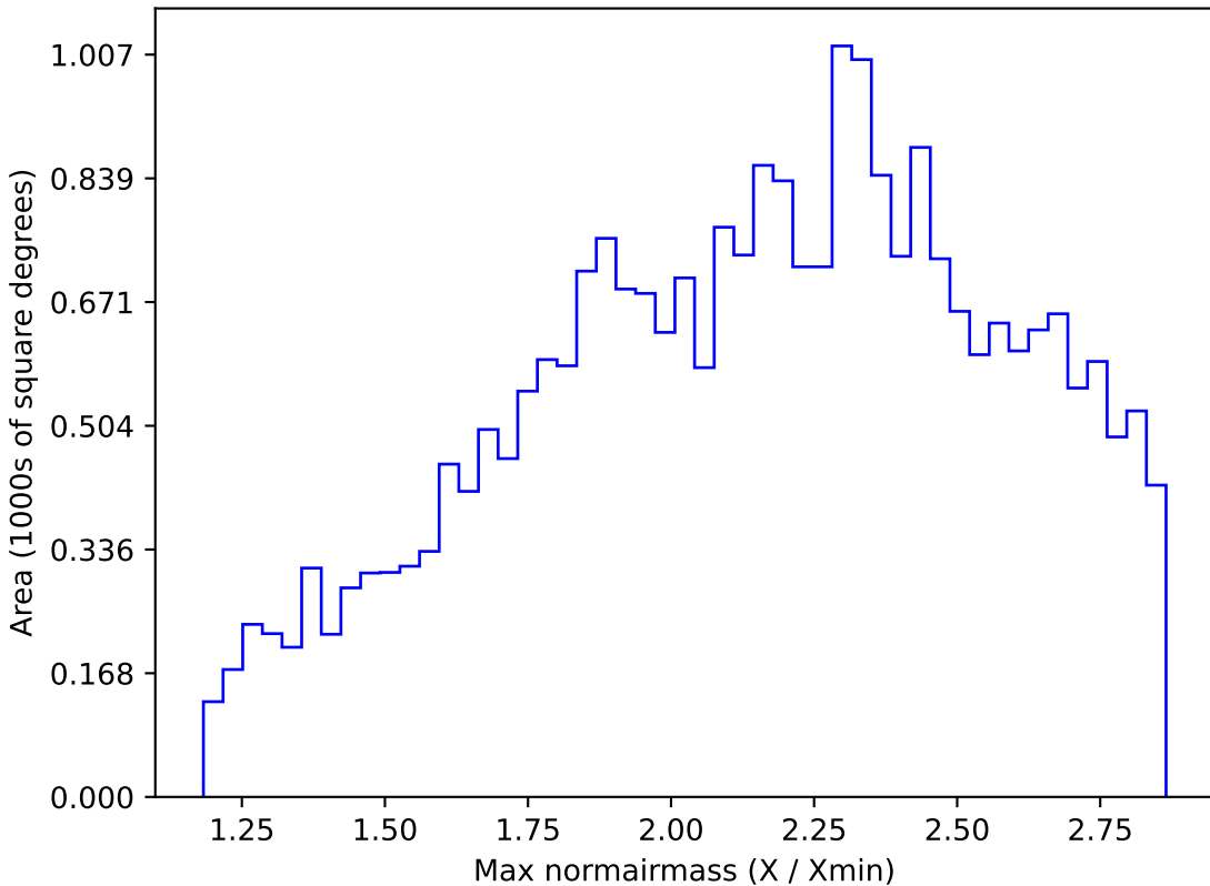
baseline_v3.3_10yrs All sky z band: Max normairmass
