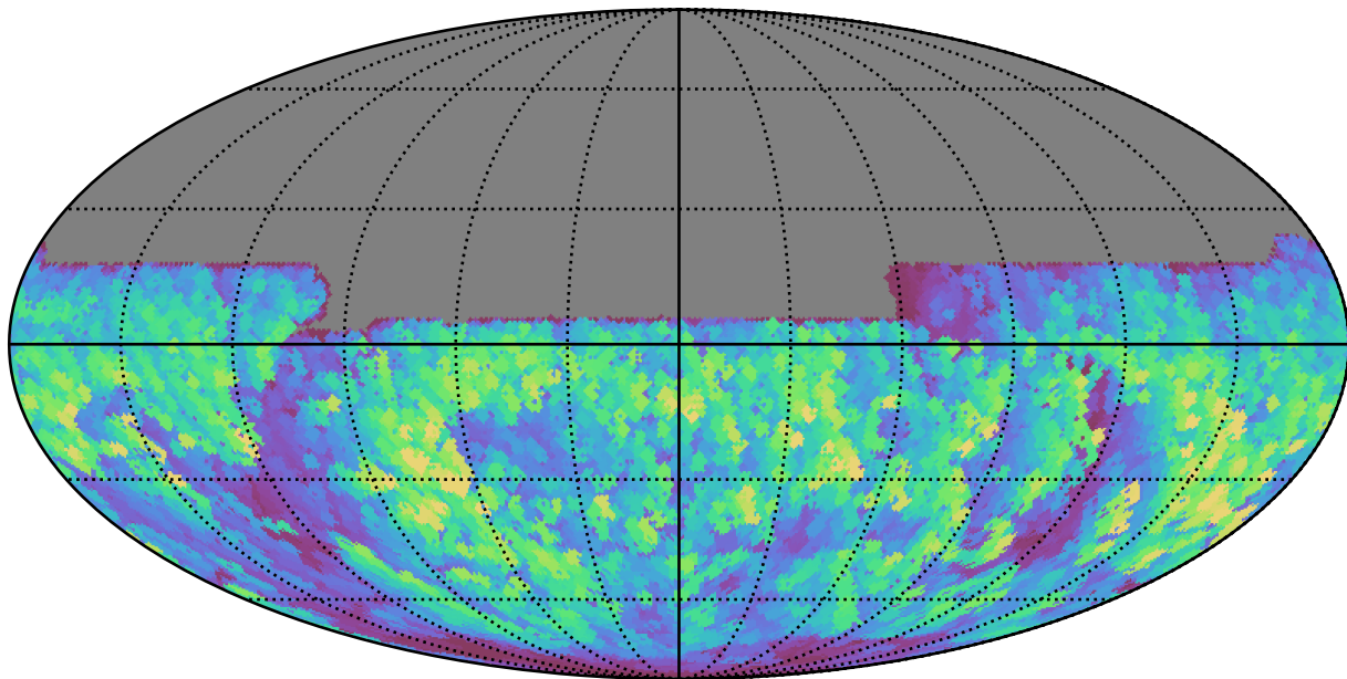
baseline_v3.3_10yrs All sky y band: Max normairmass
