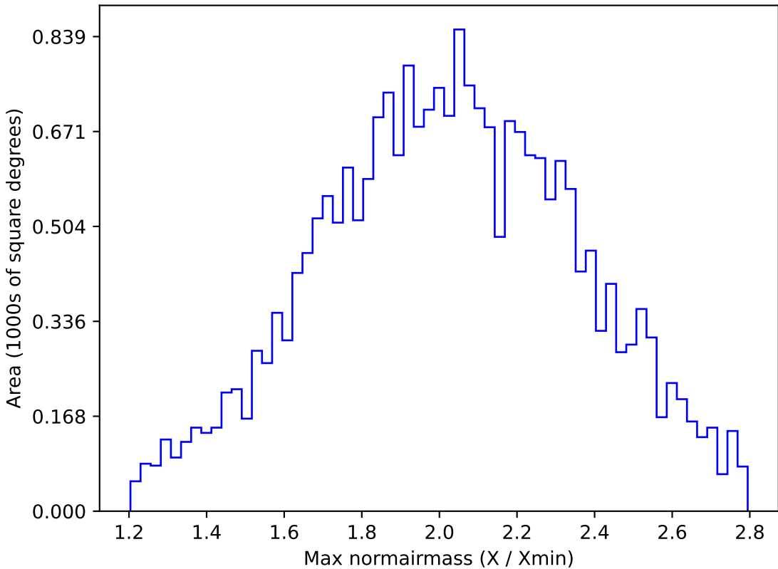
baseline_v3.3_10yrs All sky y band: Max normairmass
