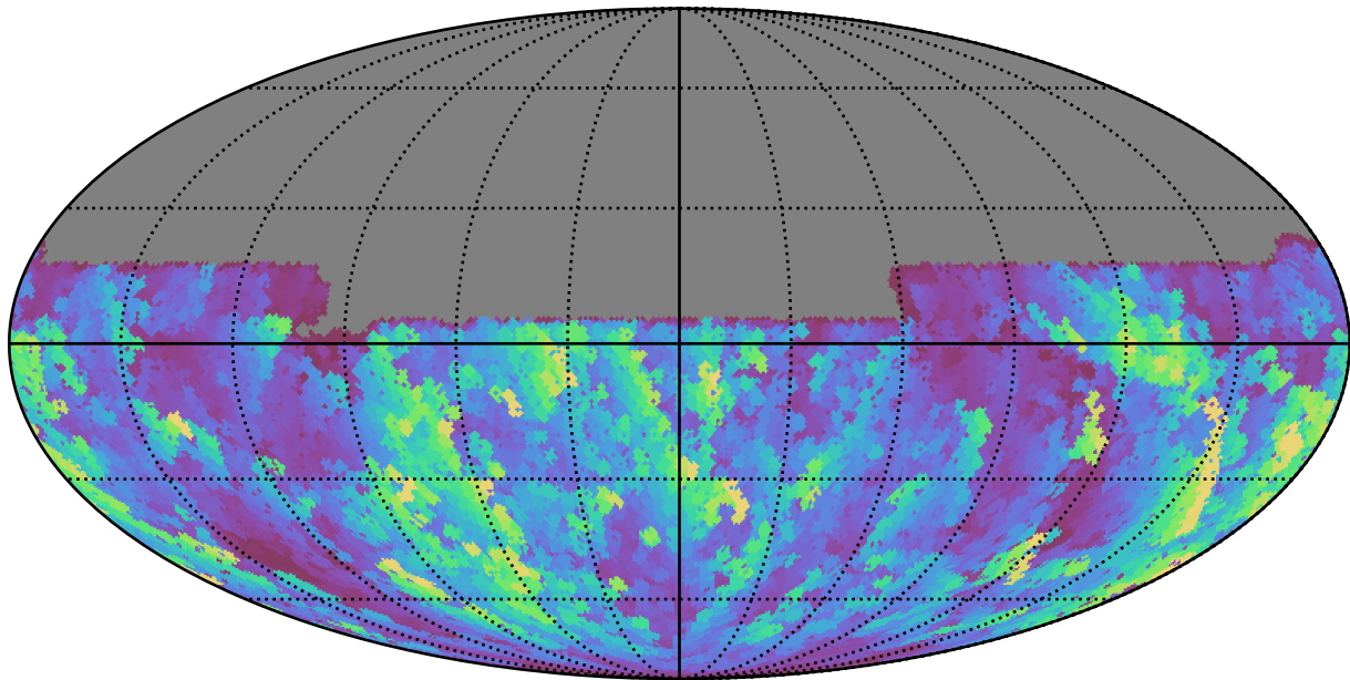
baseline_v3.3_10yrs All sky u band: Max normairmass
