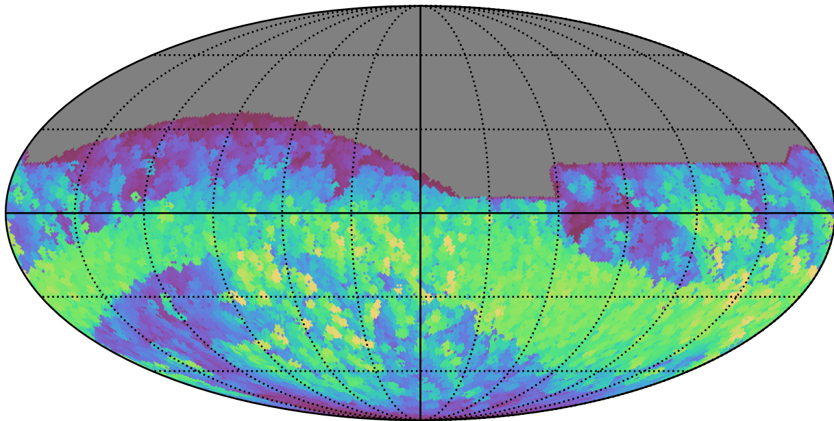
baseline_v3.3_10yrs All sky r band: Max normairmass
