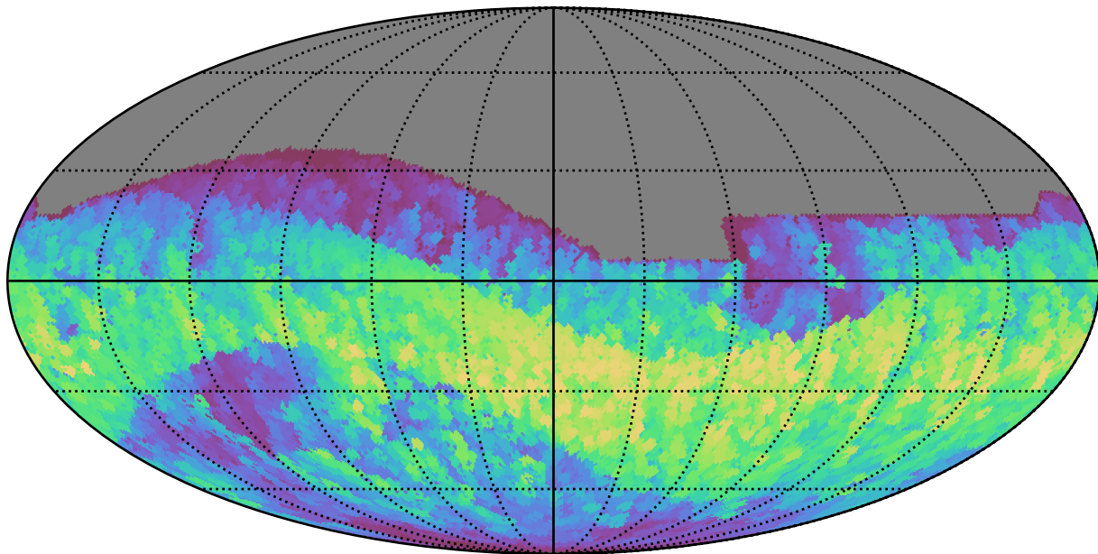
baseline_v3.3_10yrs All sky i band: Max normairmass
