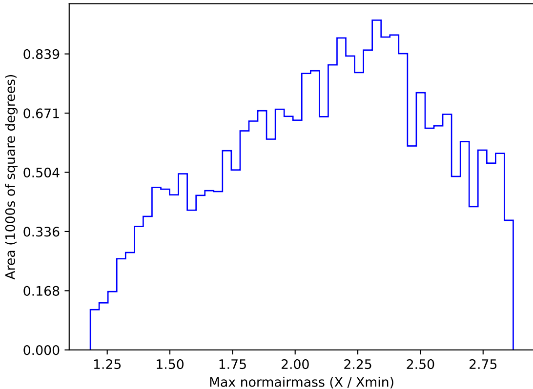
baseline_v3.3_10yrs All sky i band: Max normairmass
