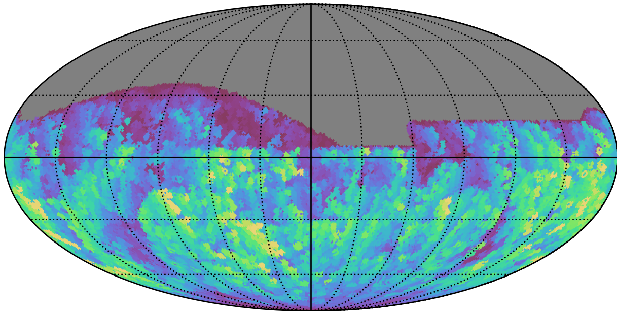
baseline_v3.3_10yrs All sky g band: Max normairmass
