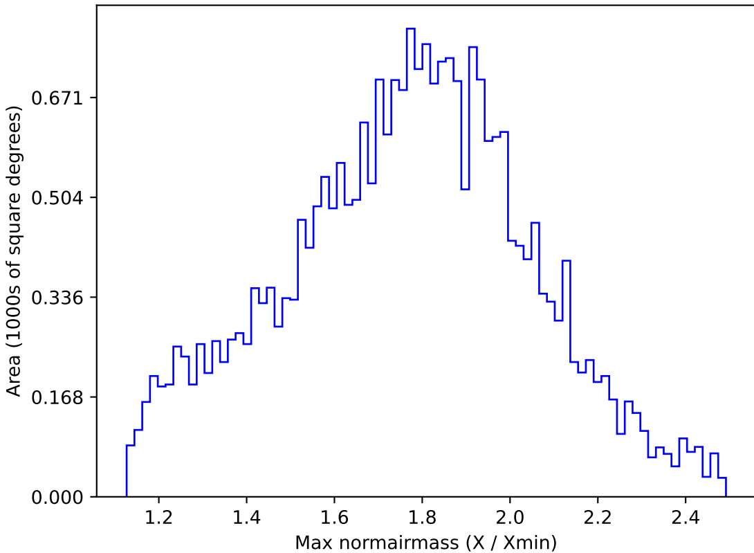
baseline_v3.3_10yrs All sky g band: Max normairmass
