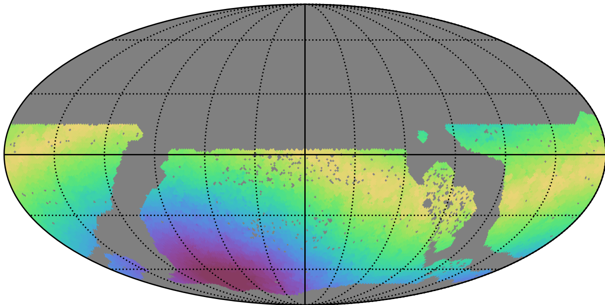
baseline_v3.3_10yrs WFD z band: Max moonDistance
