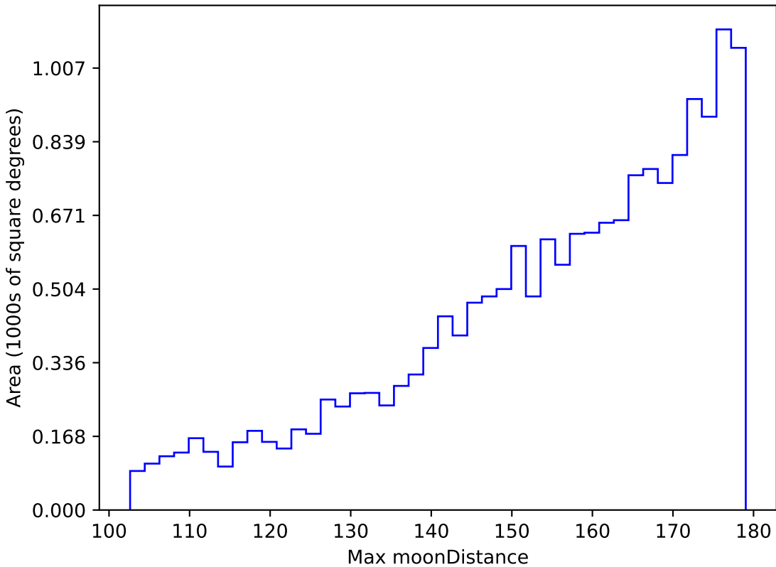
baseline_v3.3_10yrs WFD z band: Max moonDistance
