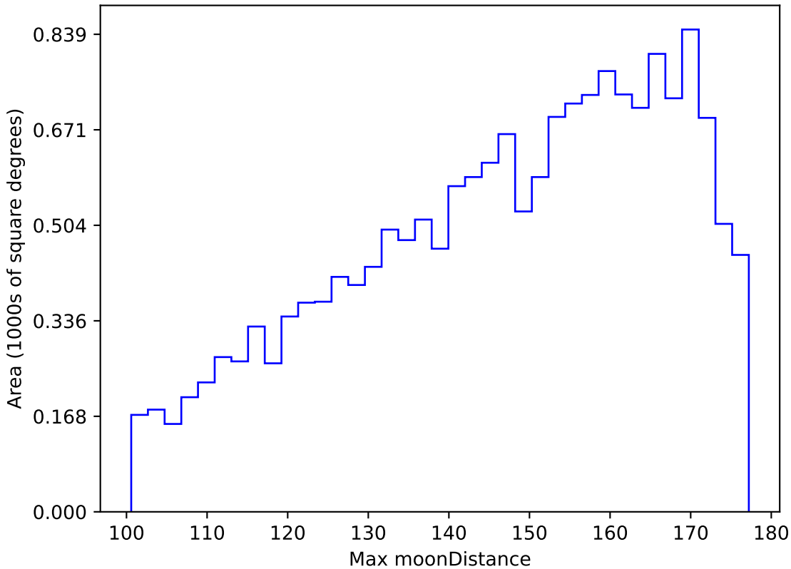
baseline_v3.3_10yrs WFD y band: Max moonDistance
