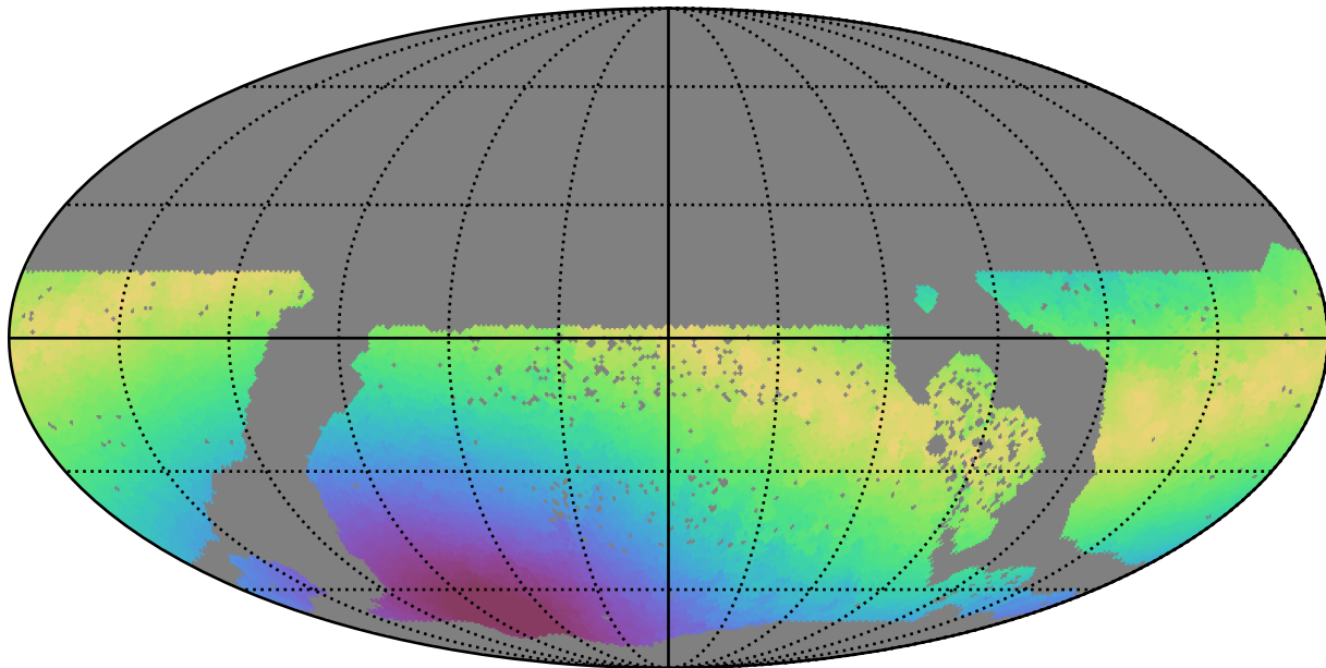
baseline_v3.3_10yrs WFD u band: Max moonDistance
