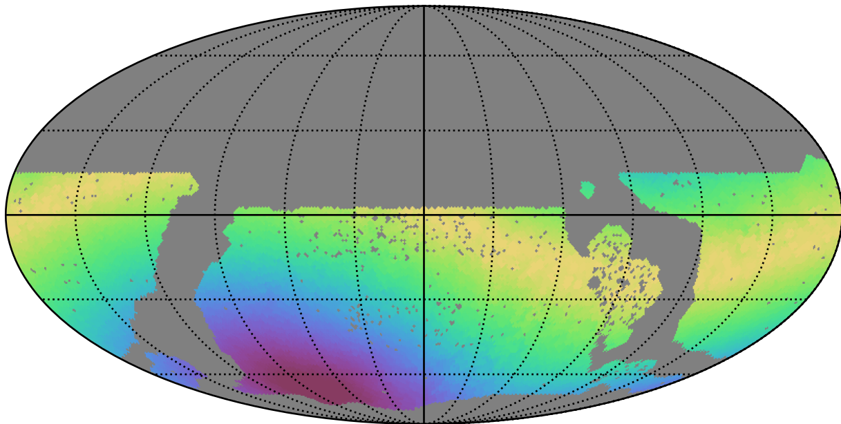
baseline_v3.3_10yrs WFD r band: Max moonDistance
