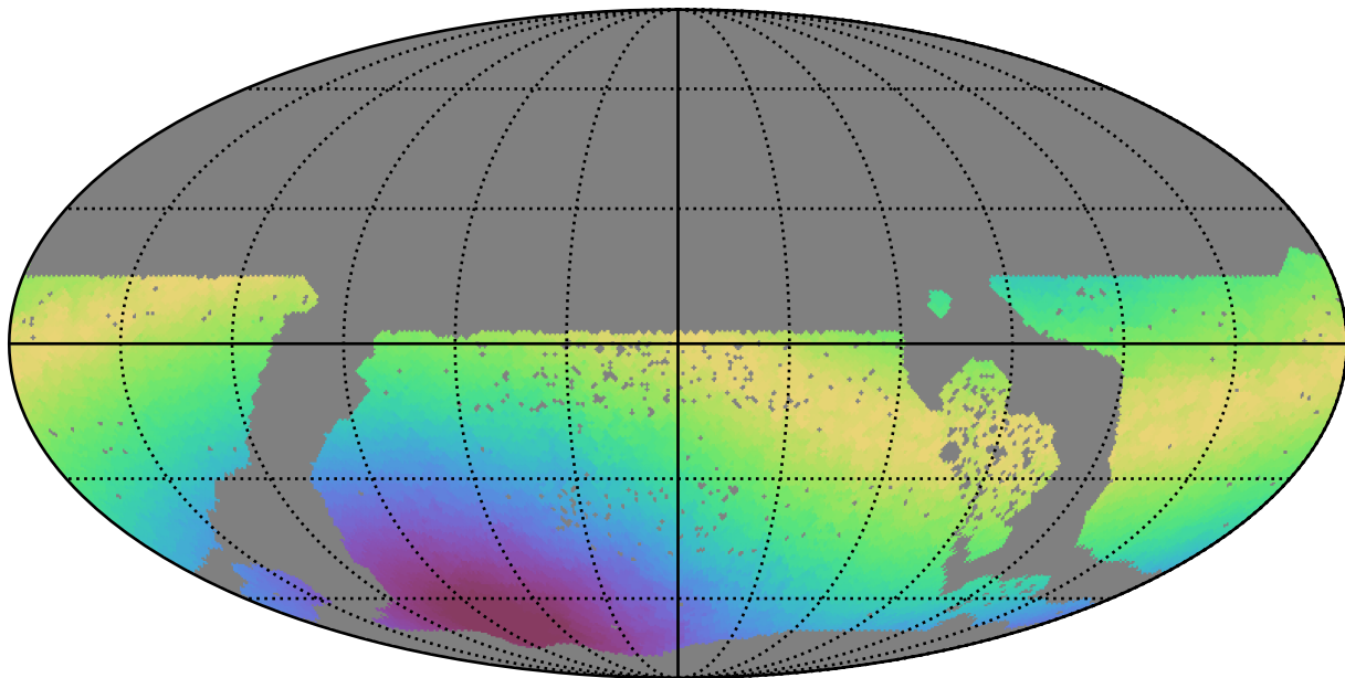
baseline_v3.3_10yrs WFD i band: Max moonDistance
