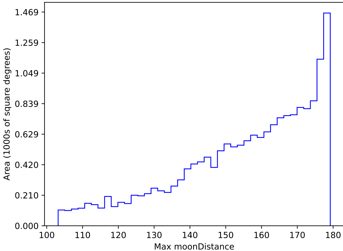
baseline_v3.3_10yrs WFD i band: Max moonDistance
