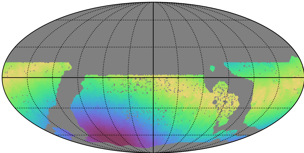
baseline_v3.3_10yrs WFD g band: Max moonDistance
