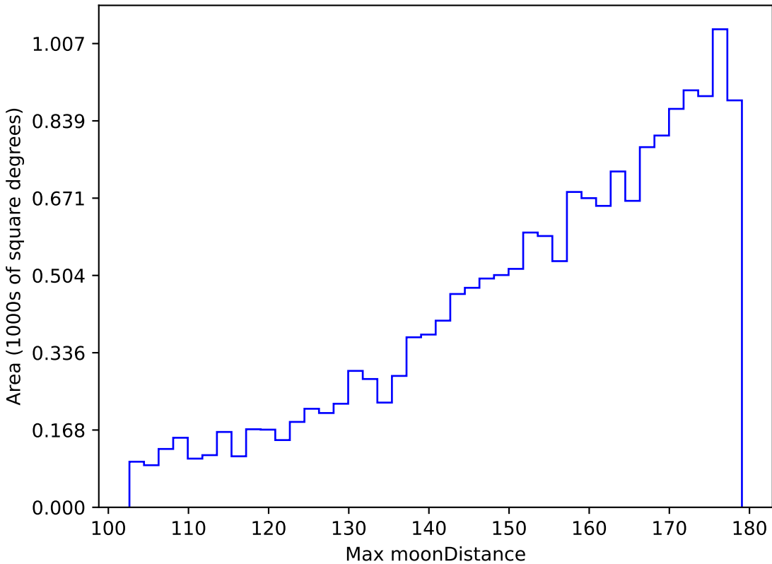
baseline_v3.3_10yrs WFD g band: Max moonDistance
