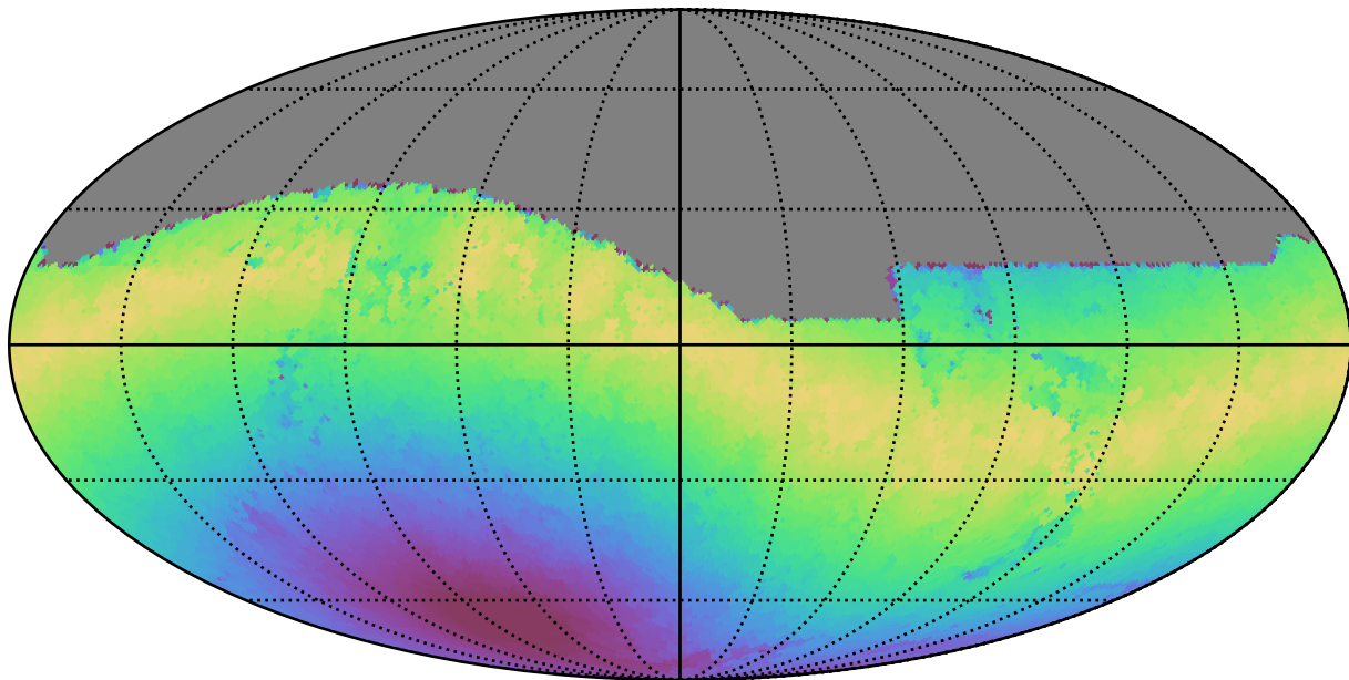
baseline_v3.3_10yrs All sky z band: Max moonDistance
