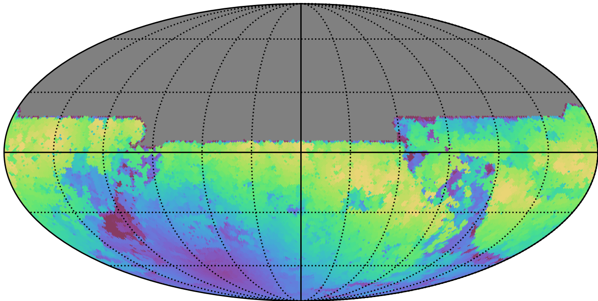
baseline_v3.3_10yrs All sky y band: Max moonDistance
