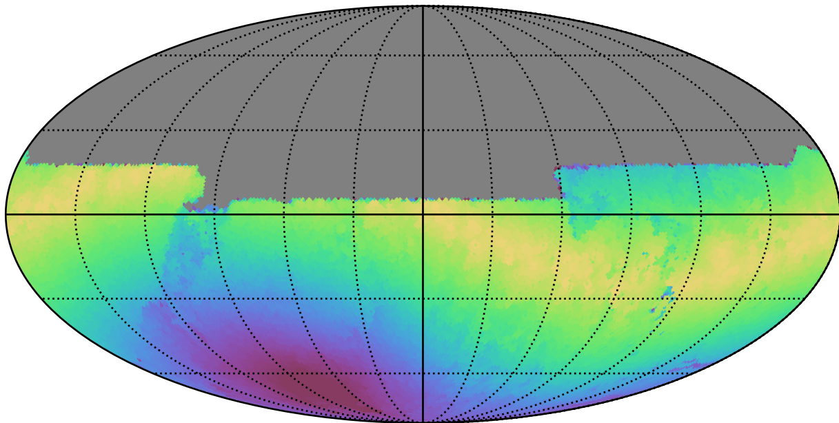
baseline_v3.3_10yrs All sky u band: Max moonDistance
