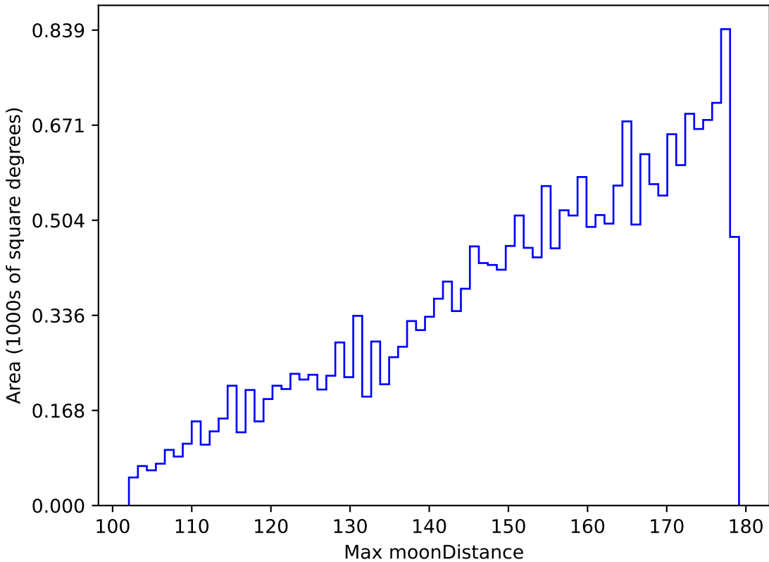
baseline_v3.3_10yrs All sky u band: Max moonDistance
