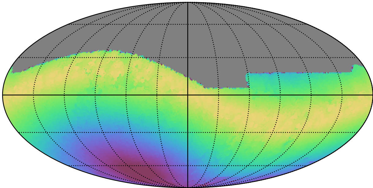
baseline_v3.3_10yrs All sky r band: Max moonDistance
