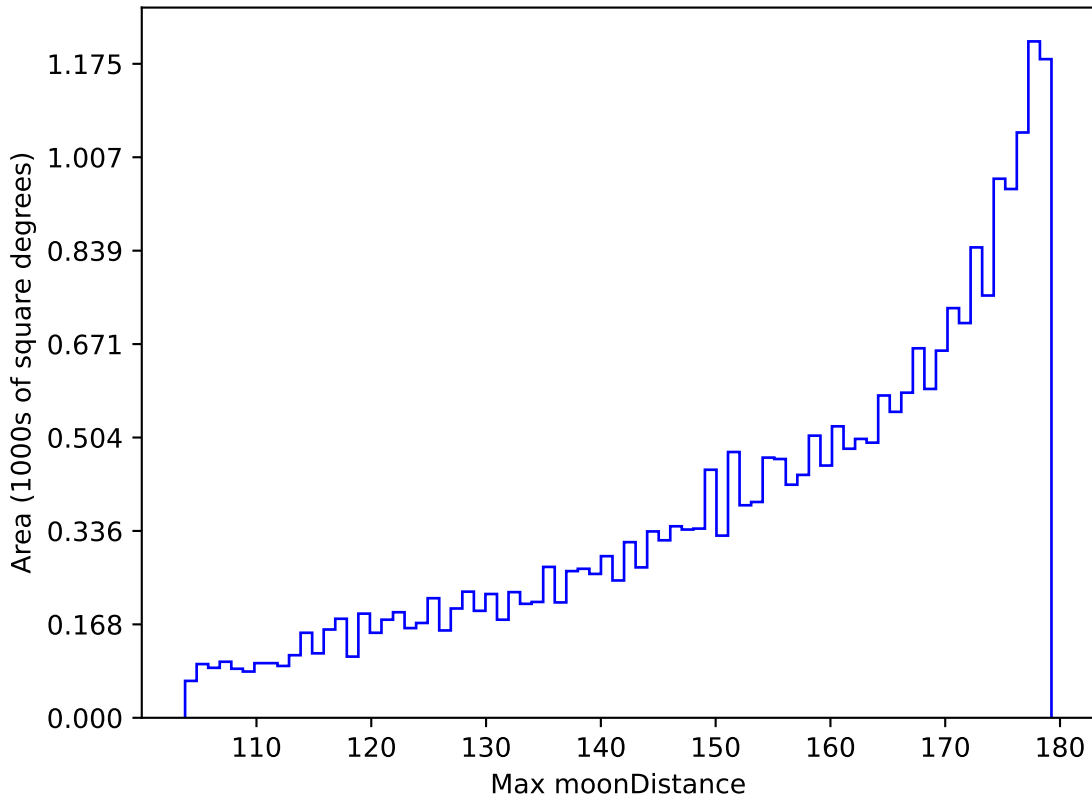
baseline_v3.3_10yrs All sky r band: Max moonDistance
