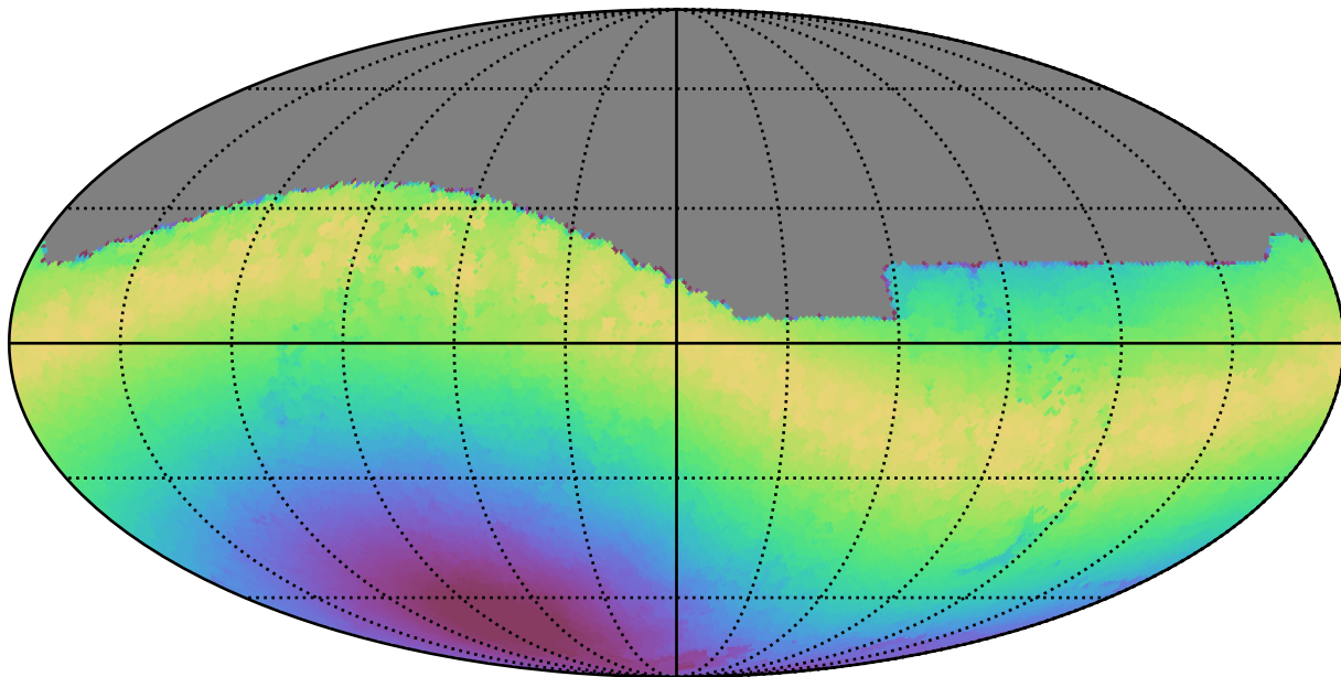
baseline_v3.3_10yrs All sky i band: Max moonDistance
