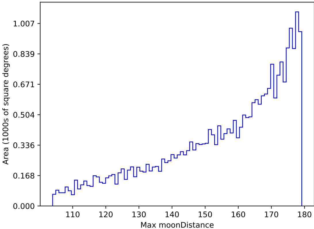
baseline_v3.3_10yrs All sky i band: Max moonDistance
