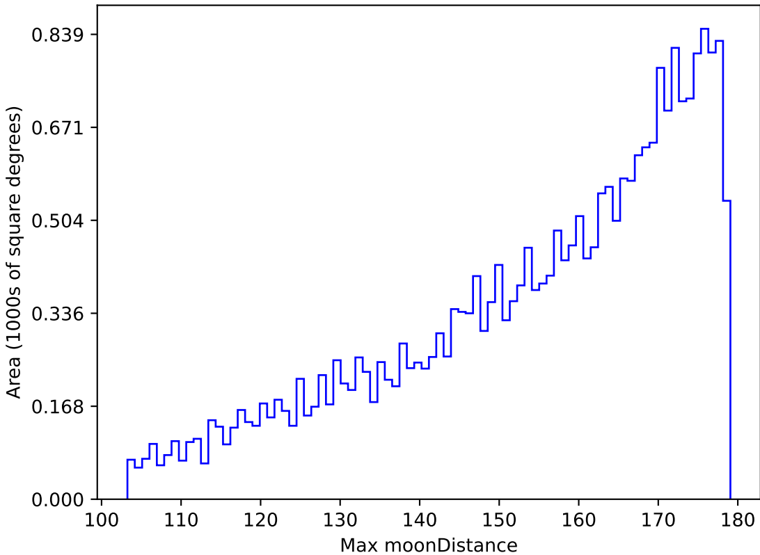
baseline_v3.3_10yrs All sky g band: Max moonDistance
