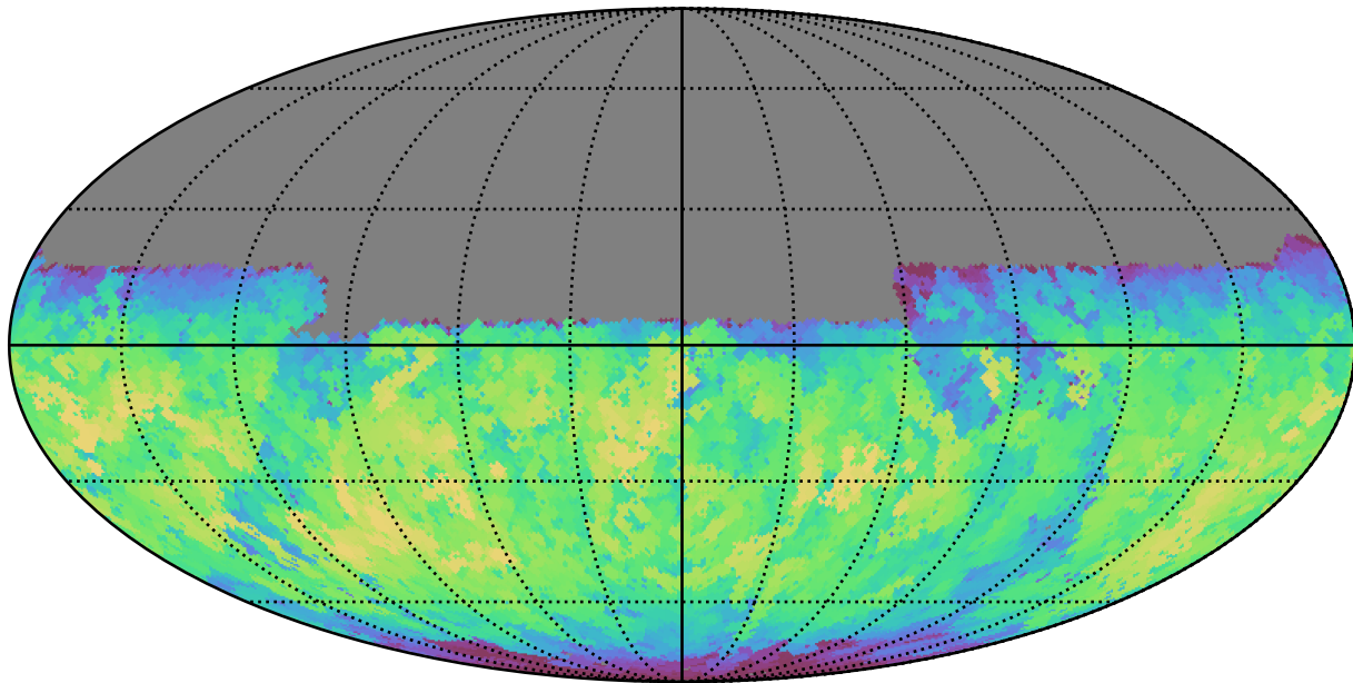
baseline_v3.3_10yrs Yr 1 y band: Max fiveSigmaDepth
