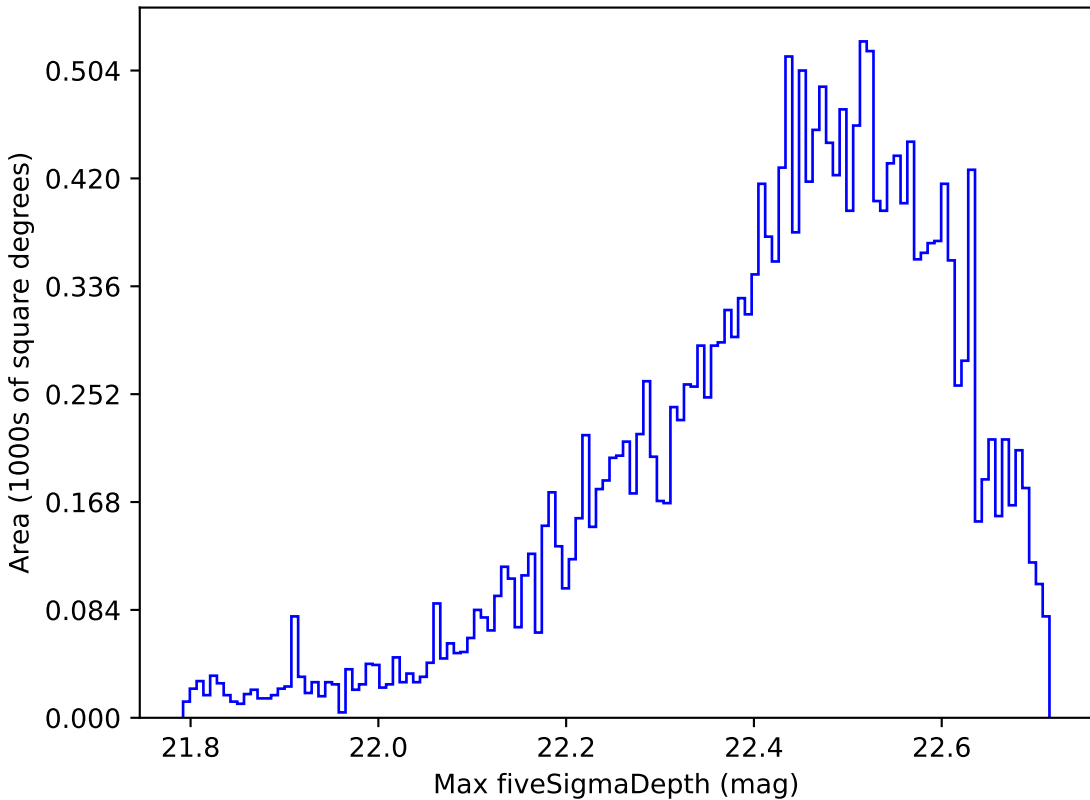
baseline_v3.3_10yrs Yr 1 y band: Max fiveSigmaDepth
