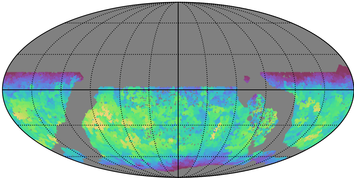
baseline_v3.3_10yrs WFD y band: Max fiveSigmaDepth
