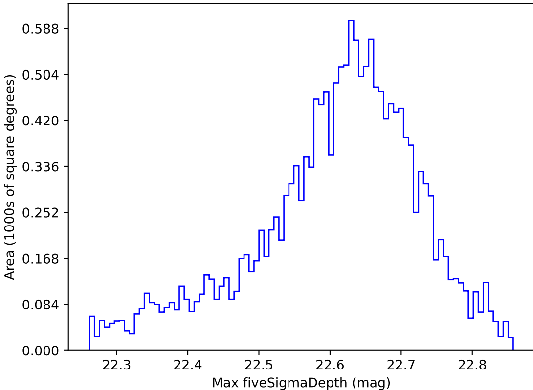
baseline_v3.3_10yrs WFD y band: Max fiveSigmaDepth
