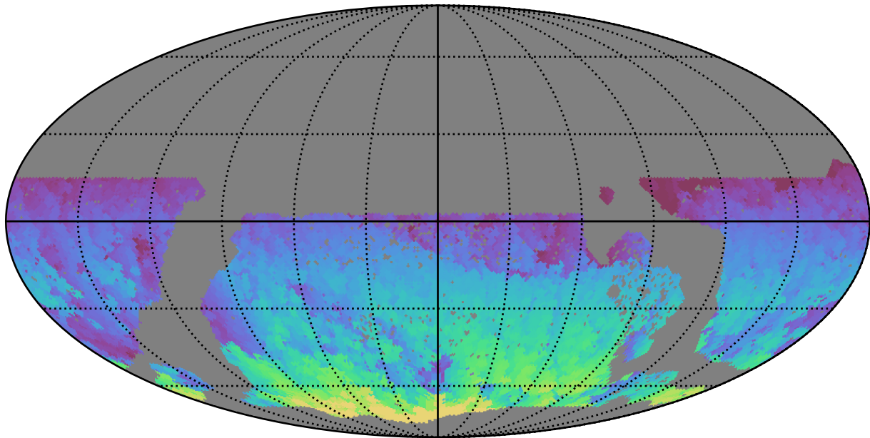
baseline_v3.3_10yrs WFD z band: Max HA
