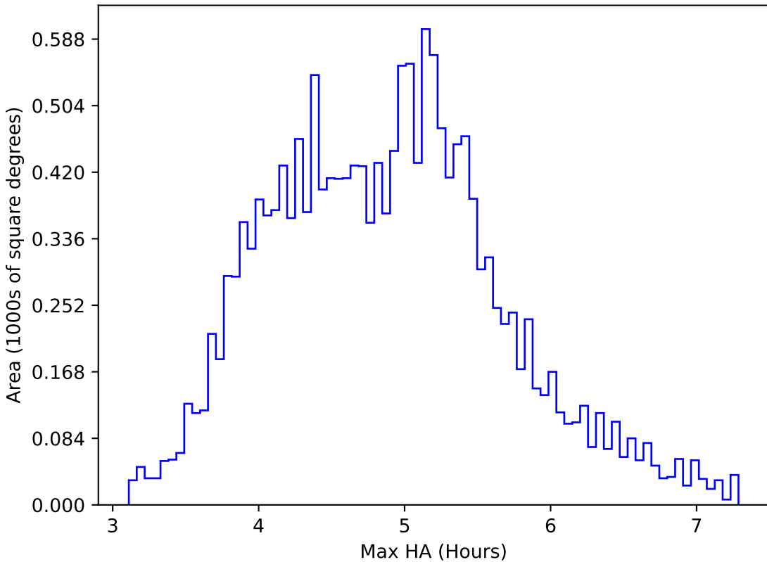
baseline_v3.3_10yrs WFD z band: Max HA
