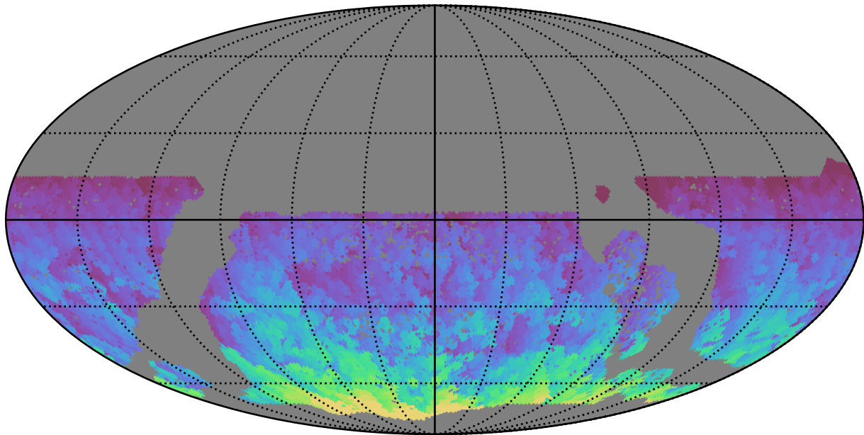
baseline_v3.3_10yrs WFD y band: Max HA
