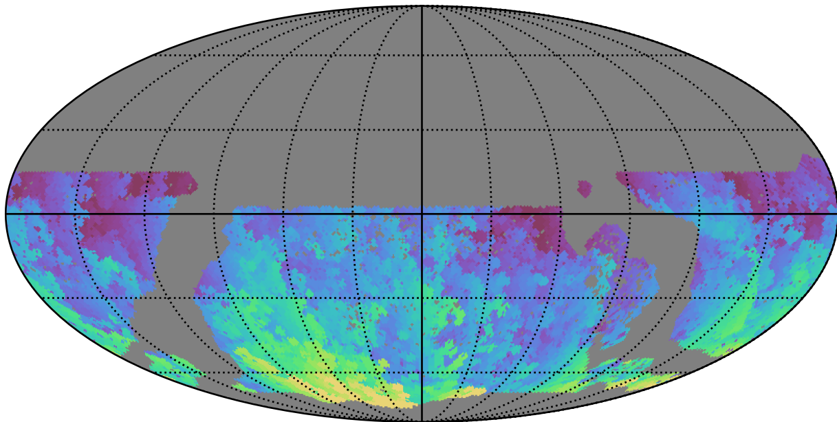
baseline_v3.3_10yrs WFD u band: Max HA
