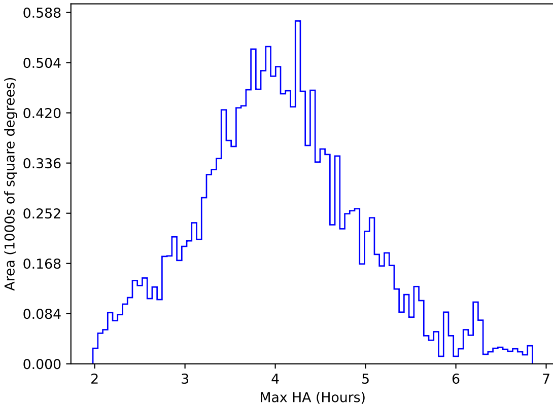
baseline_v3.3_10yrs WFD u band: Max HA
