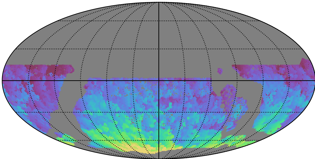
baseline_v3.3_10yrs WFD r band: Max HA
