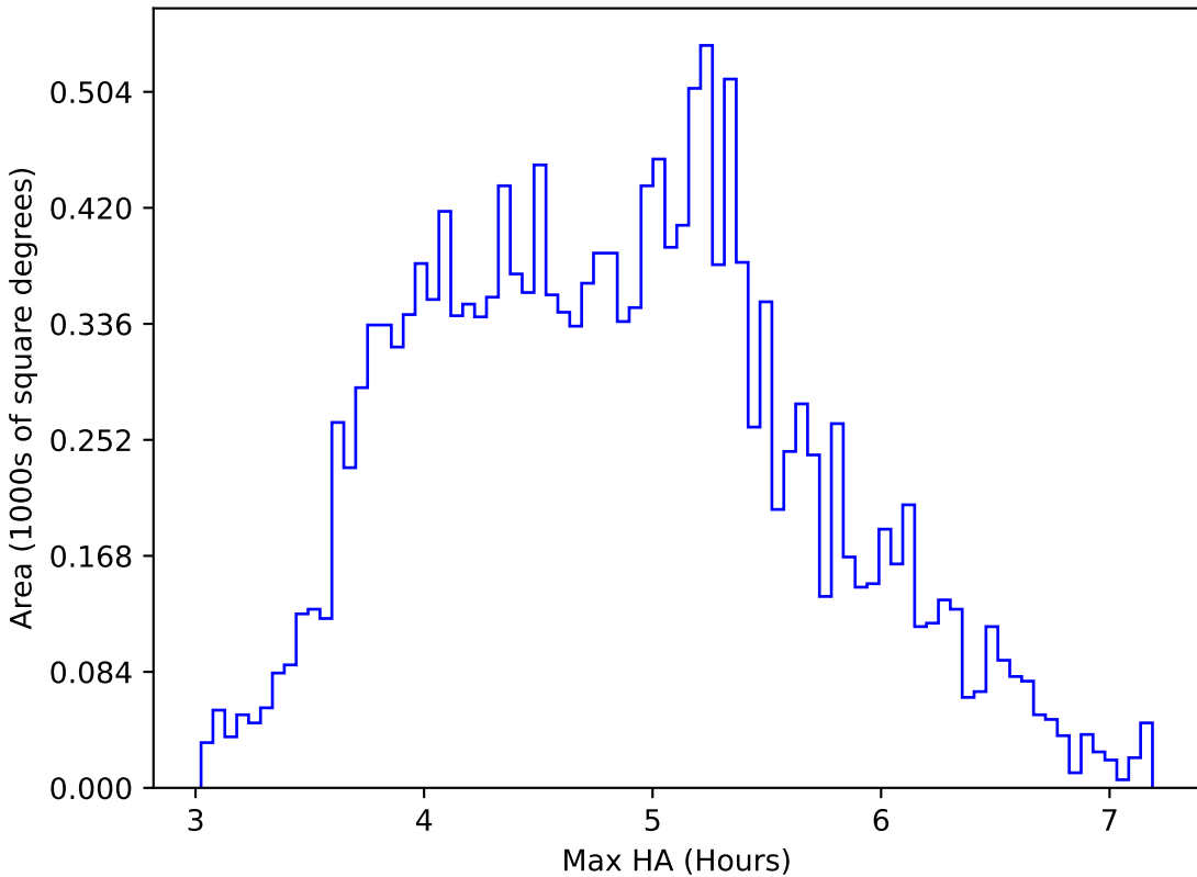
baseline_v3.3_10yrs WFD i band: Max HA
