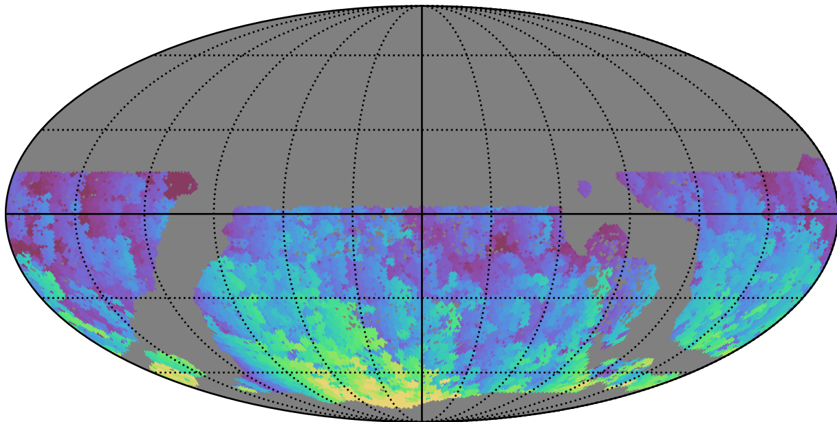
baseline_v3.3_10yrs WFD g band: Max HA
