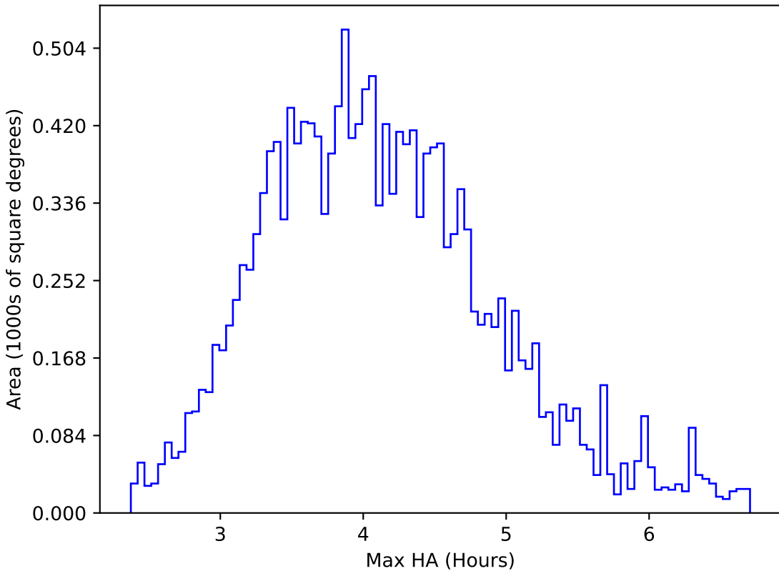
baseline_v3.3_10yrs WFD g band: Max HA
