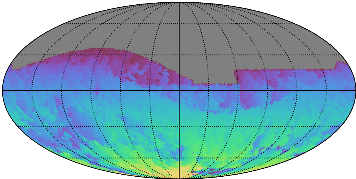
baseline_v3.3_10yrs All sky z band: Max HA
