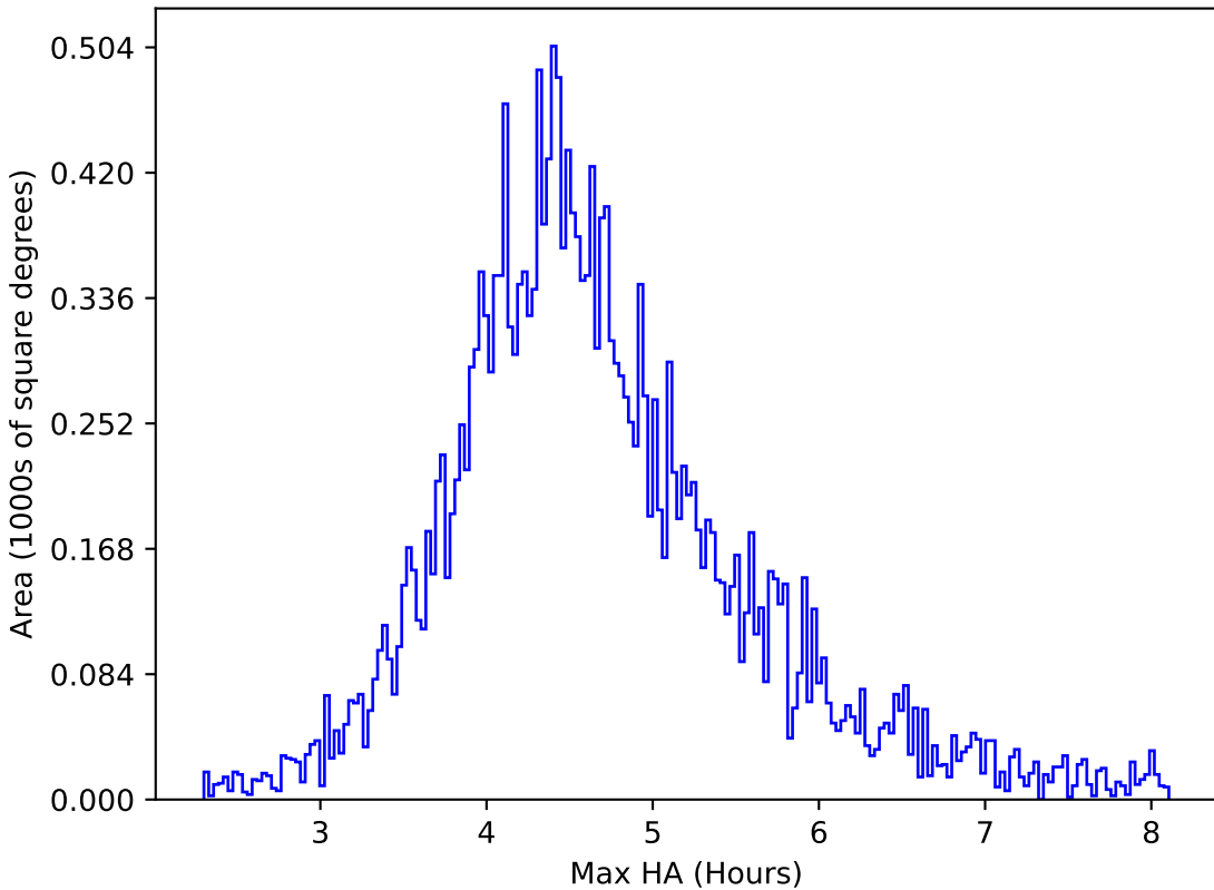
baseline_v3.3_10yrs All sky y band: Max HA
